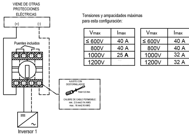
Diagrama 1. Un inversor energizado por un Seccionador SISO-40MD-B Configuración sugerida
