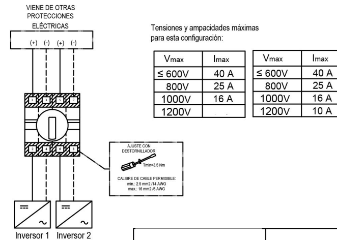
Diagrama 4. Dos inversores energizados por un Seccionador SISO-40MD-B Configuración sugerida
