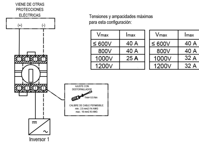
Diagrama 2. Un inversor energizado por un Seccionador SISO-40MD-B Configuración sugerida
